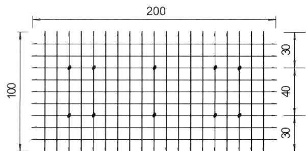
200x100x100 cm Korb Vorderansicht als Beispiel für die Lage der Distanzhalter
